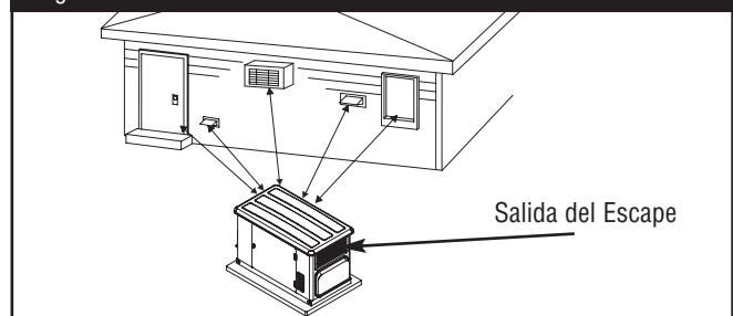
Figura 6 — Ubicación del Sistema de Generador de Doméstico
